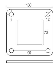
Piastra della colonna in alluminio
