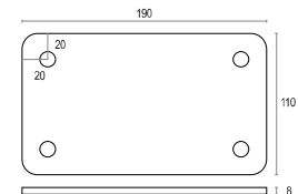
Piastra tassellare per recinzioni H 1600 - 1800 - 2000
