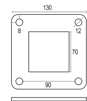
Piastra della colonna in alluminio
