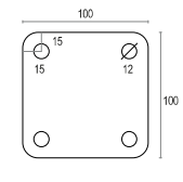
Piastra tassellare per recinzioni H 1000 - 1200 - 1400
