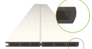
Doga terminale smussata Chiude la recinzione in altezza
