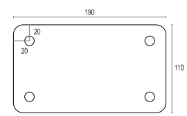
Piastra tassellare per recinzioni H 1600 - 1800 - 2000
