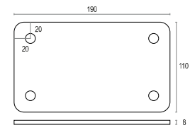
Piastra tassellare per recinzioni H 1600 - 1800 - 2000
