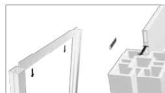
Inserire doghe "Vedo non vedo" con l'anima di rinforzo (20x10 mm zincata a freddo) inserendole dall'alto nell'incavo della colonna in WPC.
