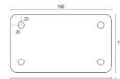
Piastra tassellare per recinzioni H 1600 - 1800 - 2000
