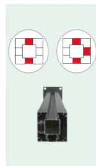
COLONNA IN ALLUMINIO COMPLETA 2 O 3 INCAVI
