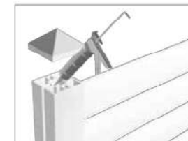
Chiudere la sommità della colonna con un tappo di chiusura con viti o colla epossidica bicomponente.
