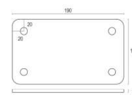
Piastra tassellare per recinzioni H 1600 - 1800 - 2000
