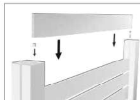
Tra una doga e l'altra vanno inseriti i distanziali infilandoli dall'alto nei canali della colonna.
