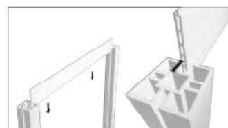
Inserire doghe "Privacy" inserendole dall'alto nell'incavo della colonna in WPC.
